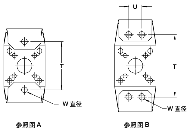
图6. 安装支架尺寸 (见表7)
