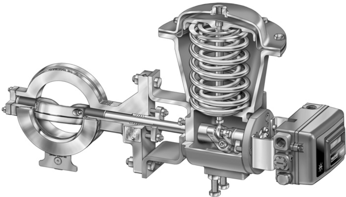
图 3. 2052 组件
