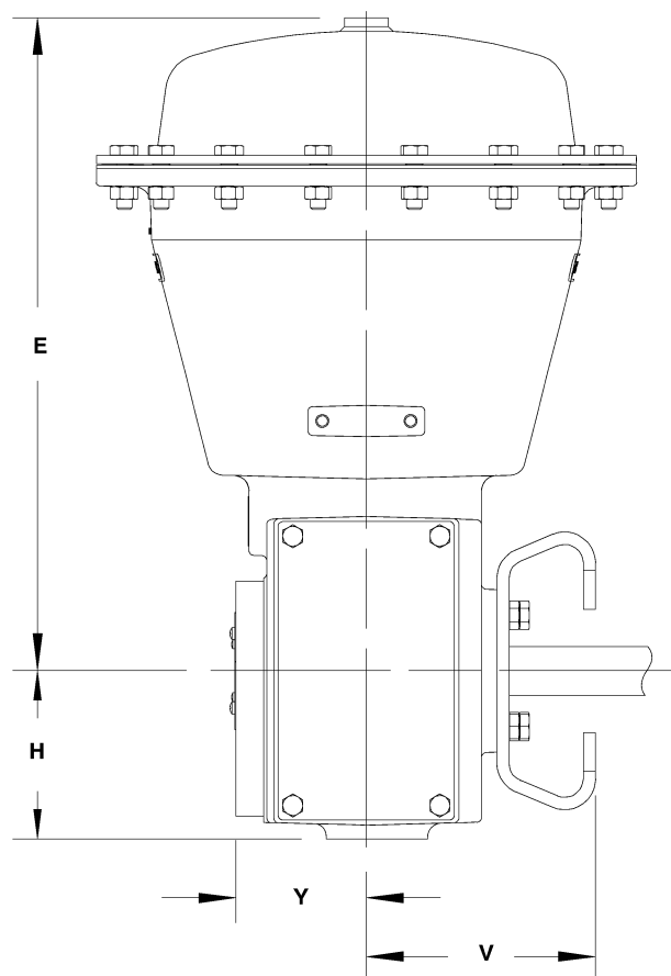
图4. 尺寸 (见表6,7和8)
