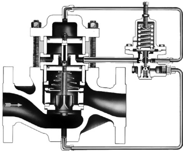
配有6492H型指挥器的 2英寸(DN 50)主阀
