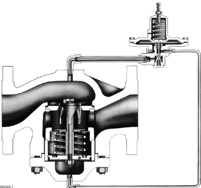
配有WHIPSER TRIM噪声衰减器和6492L型指挥器的 4英寸(DN 100)主阀
